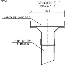
SUMIDERO (COTAS EN mm.)
