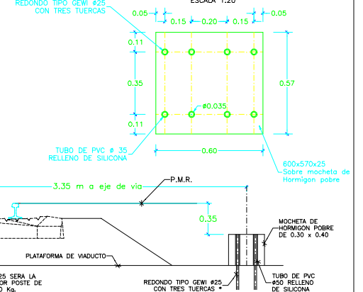
PLACA CATENARIA ESCALA 1:20
