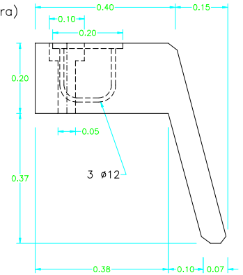
PLACA CATENARIA ESCALA 1:20
