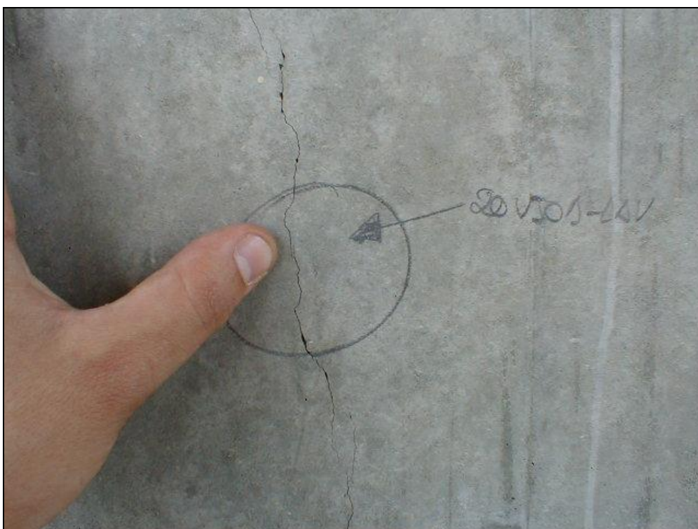
Foto 10: Fisuras en estribos
