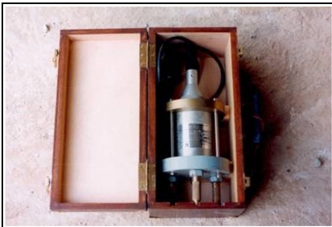
Foto 10: Sismómetro
