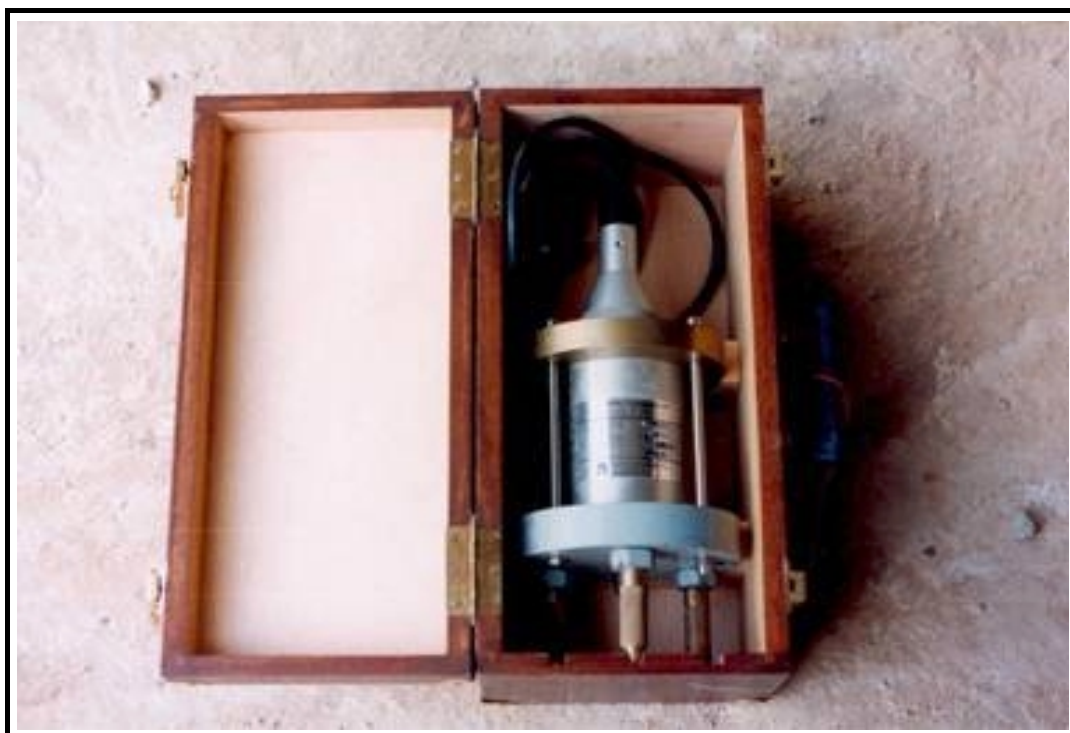
Foto 8: Sismómetro
