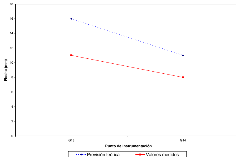
04PI06. Marco vía 2 Reparto transversal en ensayo estático para valores de deformación unitaria
