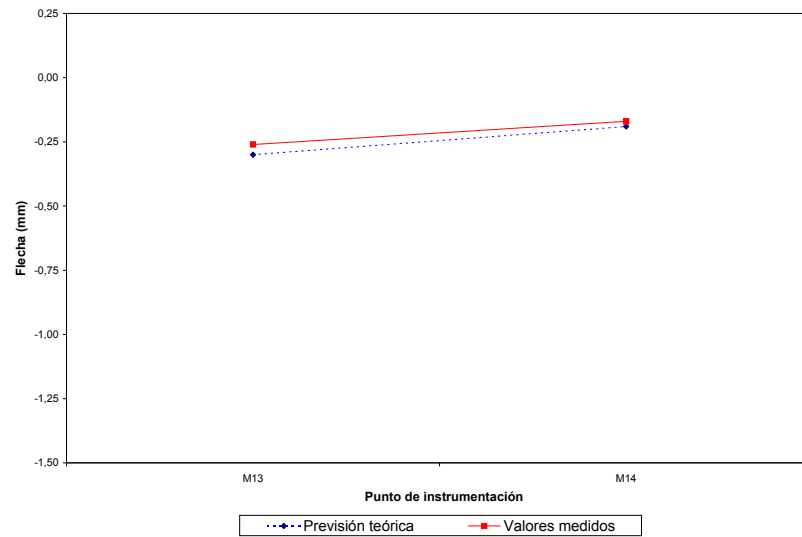
04PI06. Marco vía 2 Reparto transversal en ensayo estático para valores de flecha
