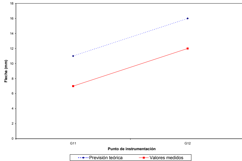
04PI06. Marco vía 1 Reparto transversal en ensayo estático para valores de deformación unitaria
