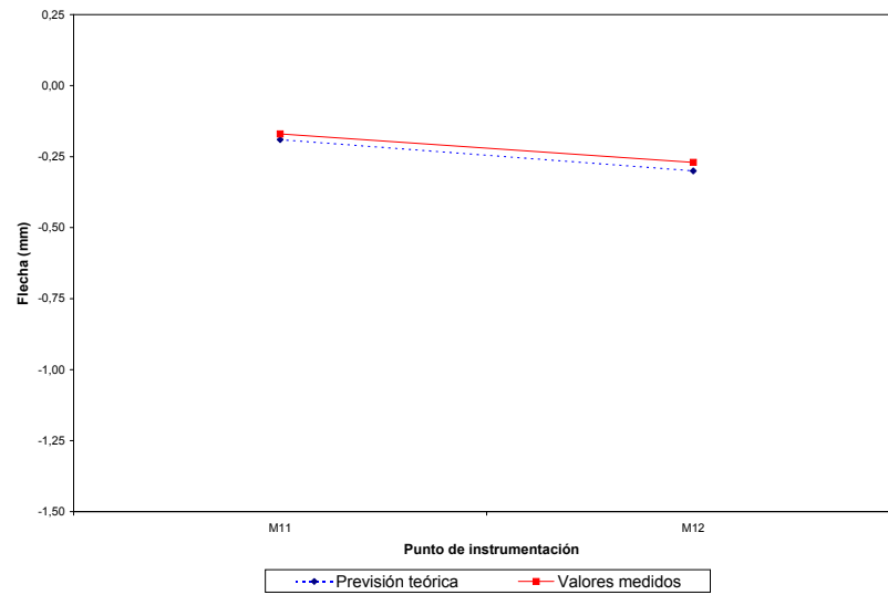
04PI06. Marco vía 1 Reparto transversal en ensayo estático para valores de flecha
