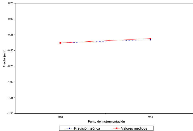
04PI04. Marco vía 2 Reparto transversal en ensayo estático para valores de flecha
