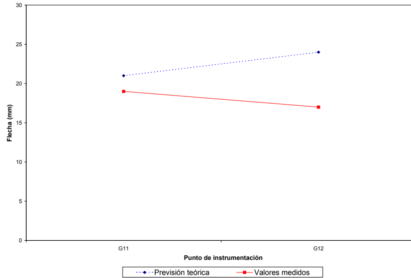
04PI04. Marco vía 1 Reparto transversal en ensayo estático para valores de deformación unitaria
