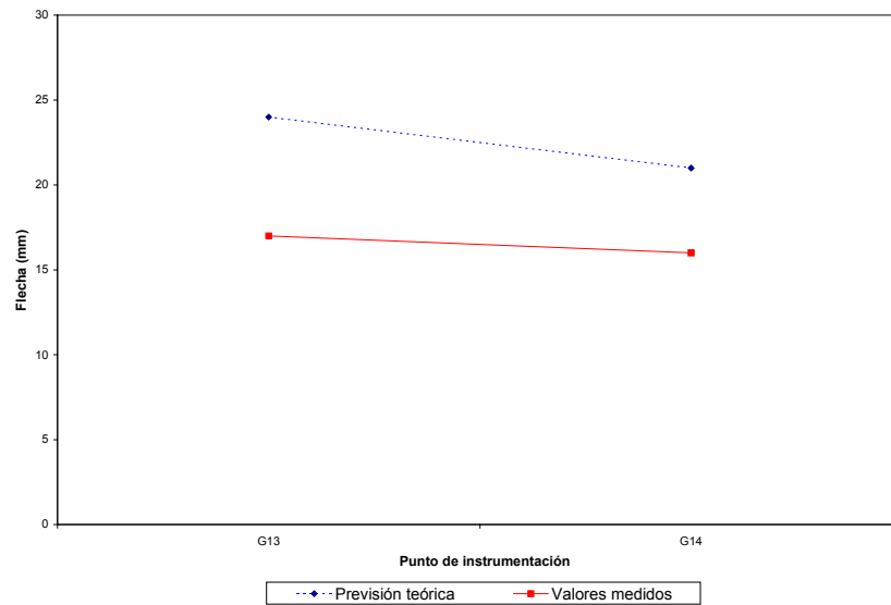
04PI04. Marco vía 2 Reparto transversal en ensayo estático para valores de deformación unitaria
