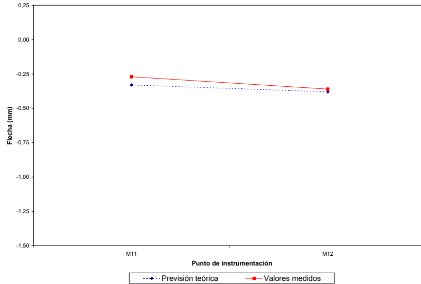
04PI04. Marco vía 1 Reparto transversal en ensayo estático para valores de flecha
