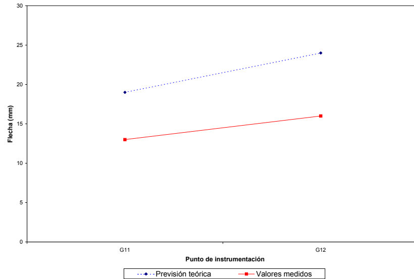
04PI03. Marco vía 1 Reparto transversal en ensayo estático para valores de deformación unitaria
