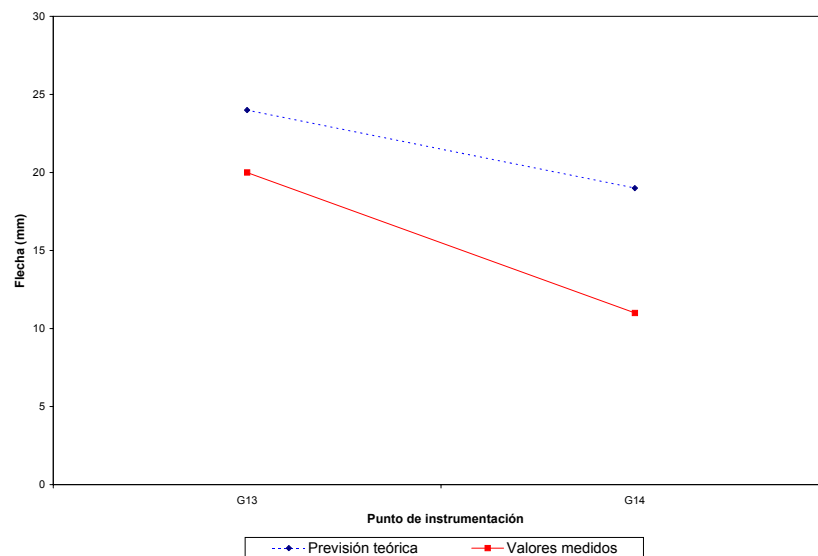
04PI03. Marco vía 2 Reparto transversal en ensayo estático para valores de deformación unitaria
