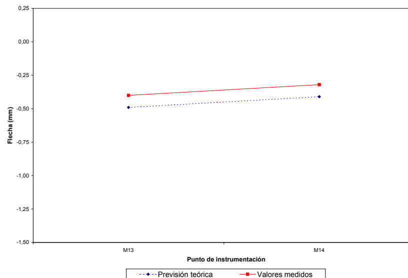
04PI03. Marco vía 2 Reparto transversal en ensayo estático para valores de flecha
