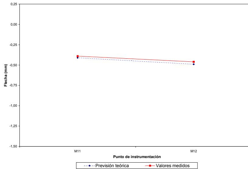
04PI03. Marco vía 1 Reparto transversal en ensayo estático para valores de flecha
