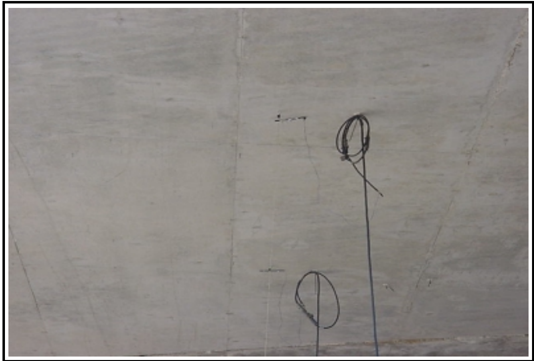
Foto 6: Bandas extensométricas en centro de vano
