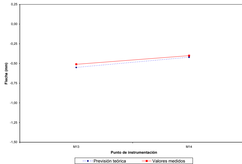
04PI02. Marco vía 2 Reparto transversal en ensayo estático para valores de flecha
