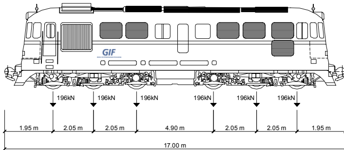
Locomotora 060
