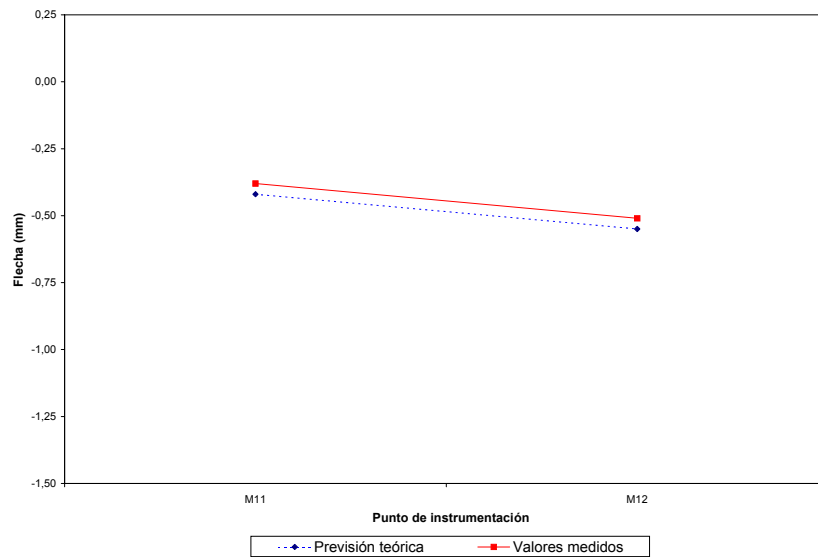
04PI02. Marco vía 1 Reparto transversal en ensayo estático para valores de flecha
