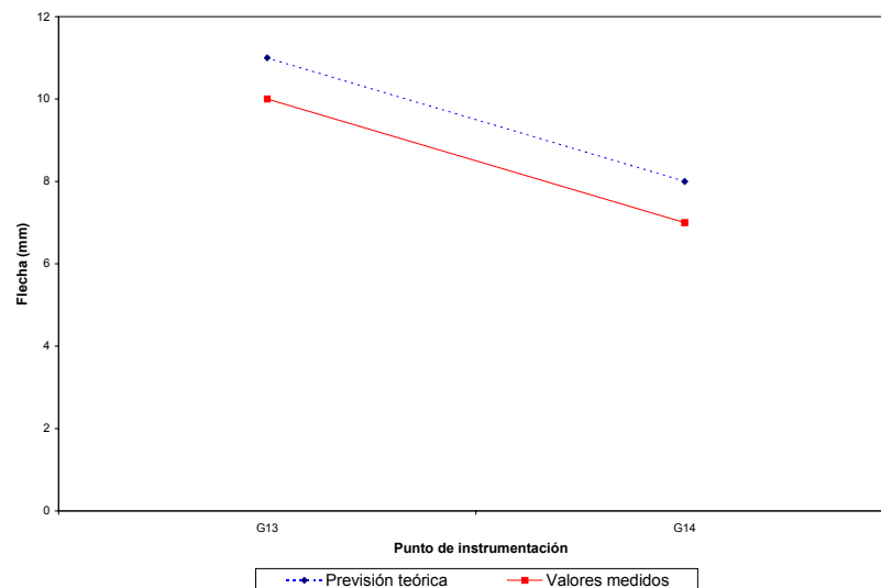
04PI01. Marco vía 2 Reparto transversal en ensayo estático para valores de deformación unitaria
