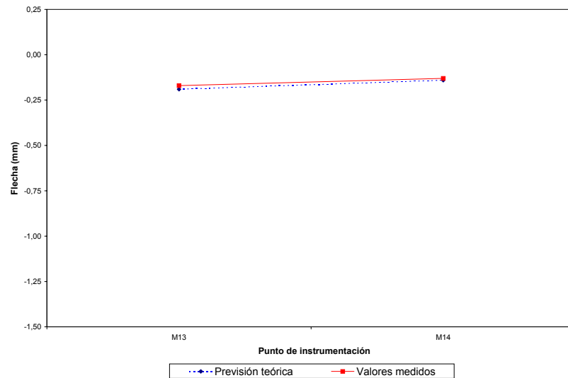
04PI01. Marco vía 2 Reparto transversal en ensayo estático para valores de flecha
