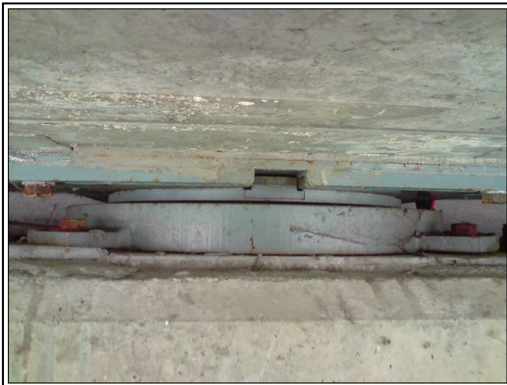
Apoyo izquierdo de estribo uno.
