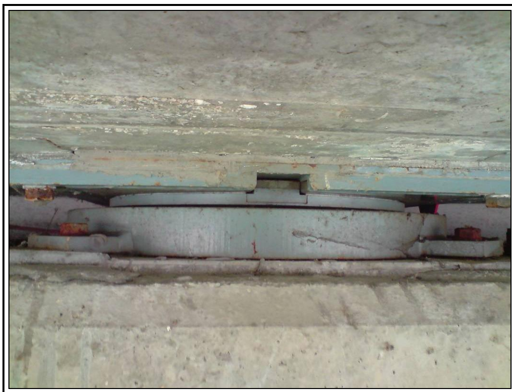
Falta de contacto de apoyo con cama de nivelación.
