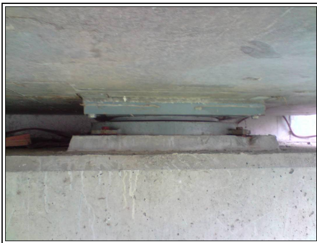
Desconchón en cama de nivelación próximo a perno.
