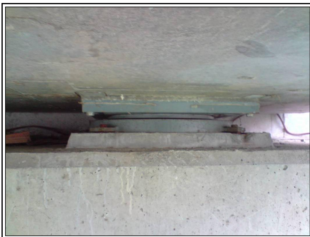
Apoyo derecho de estribo uno.
