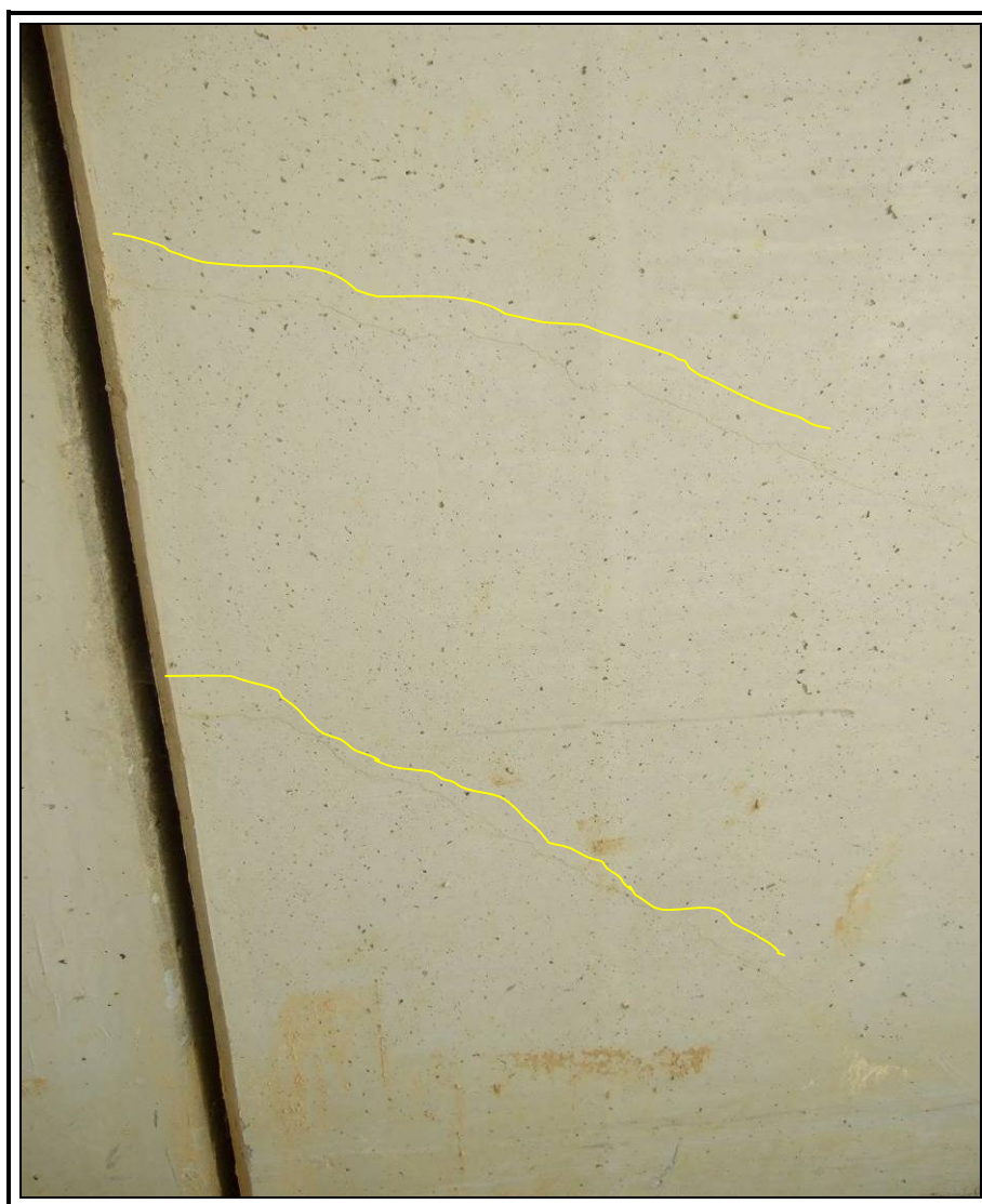
Familia de fisuras en elemento del decimoctavo anillo del estribo 1 lado izquierdo.
