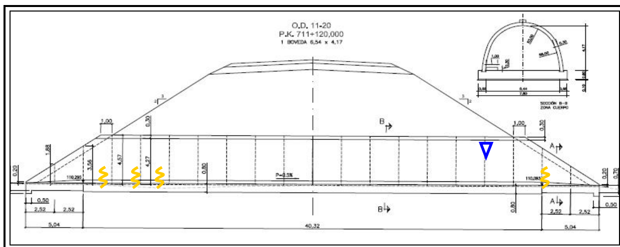
Alzado y sección.
