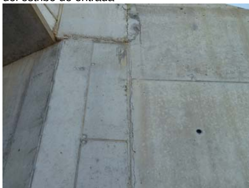
Fotografía nº 9. Fisuras en la aleta izquierda del estribo de entrada
