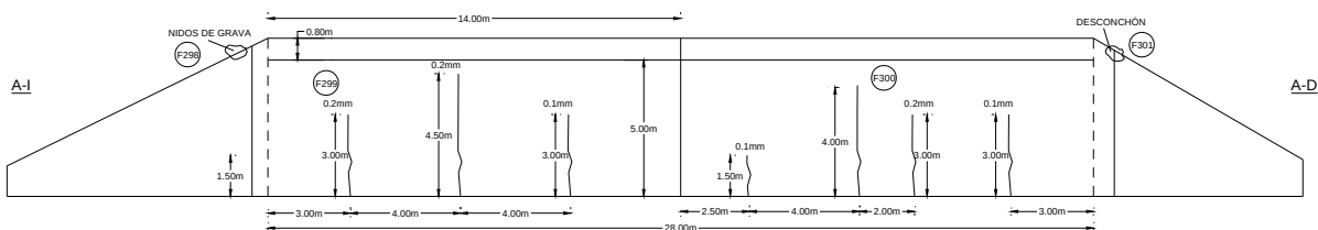
Croquis nº 2. Estribo de salida
