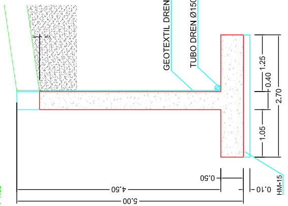
SECCIÓN E-E ESCALA 1:60
