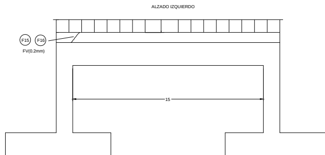
Croquis nº 3. Paramento inferior de la losa superior
