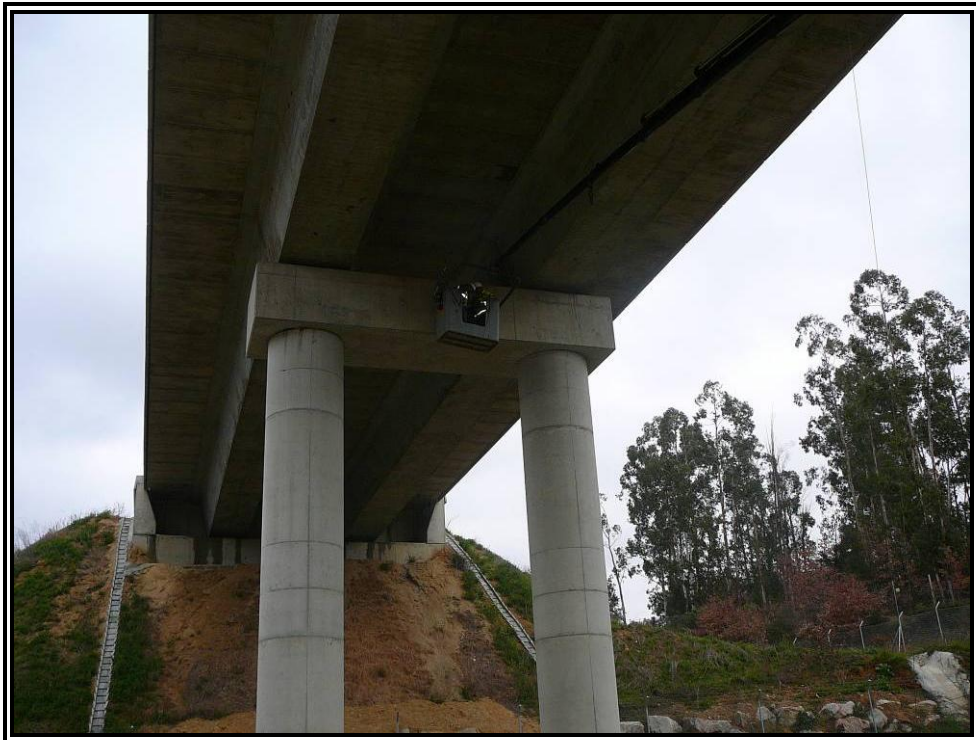
Nº 7.- Colocación de instrumentación en apoyo.
