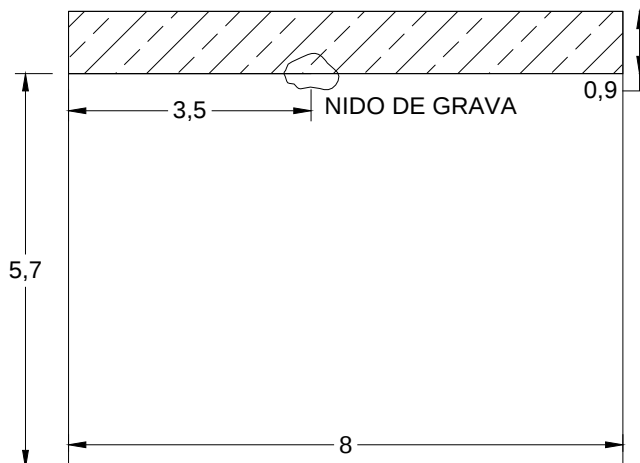
Croquis nº 3. Paramento inferior de la losa superior
