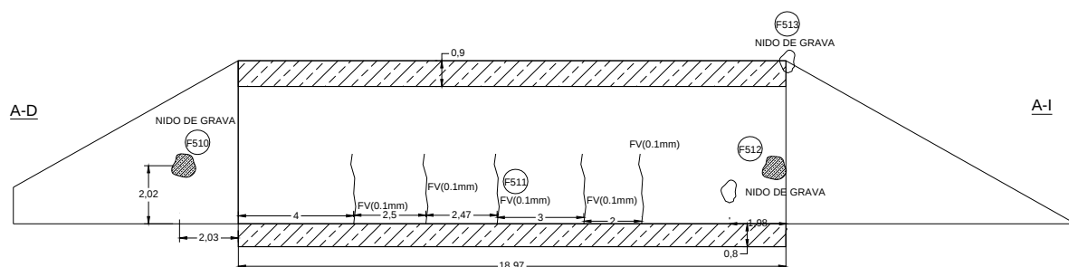
Croquis nº 1. Estribo de entrada
