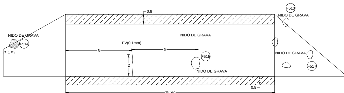
Croquis nº 2. Estribo de salida
