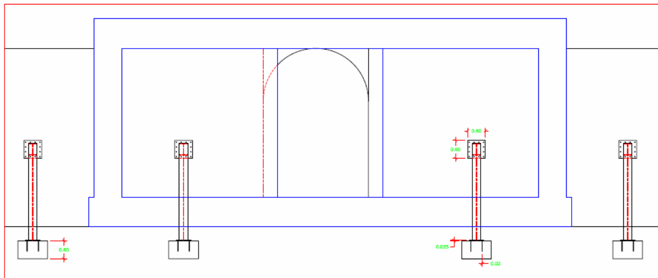
ALZADO ESCALA 1:75
