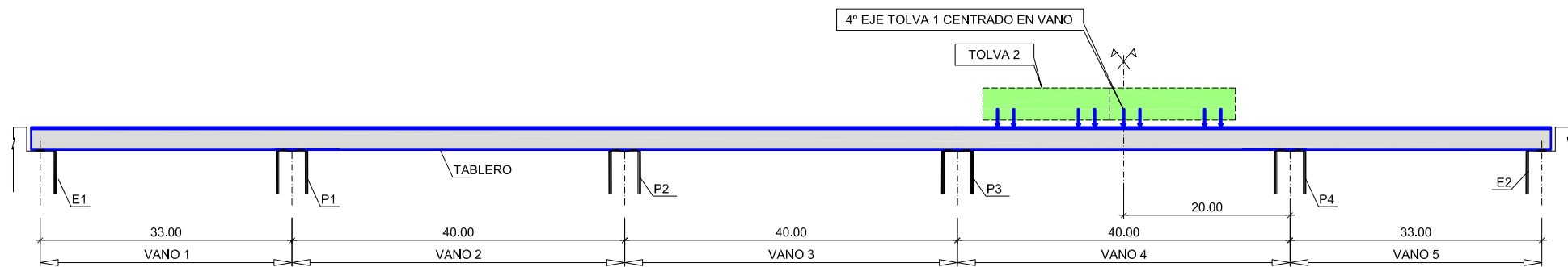
ALZADO
