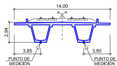
SECCIÓN TRANSVERSAL
