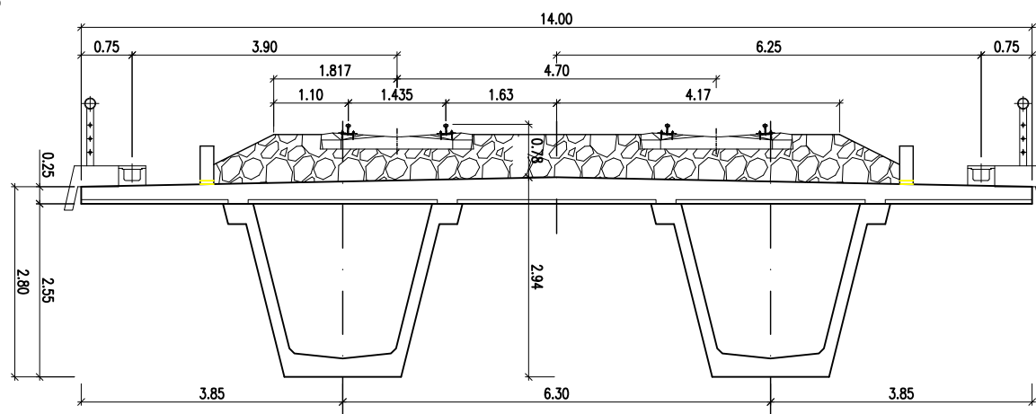
SECCIÓN TIPO ESCALA 1/100
