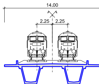
SECCIÓN TRANSVERSAL
