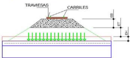
Figura 1-c: Sección transversal
