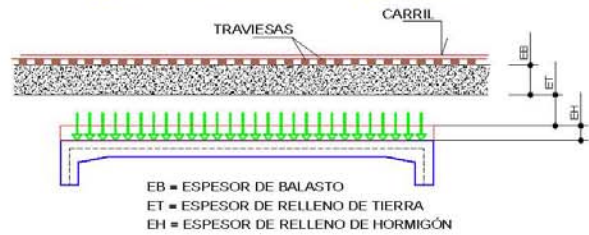
Figura 1-b: sección Longitudinal
