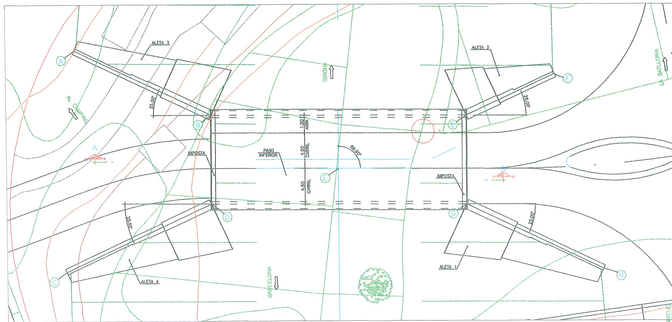
PLANTA ESCALA 1/200
