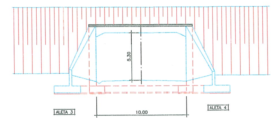
VISTA POR -C- ESCALA 1/250
