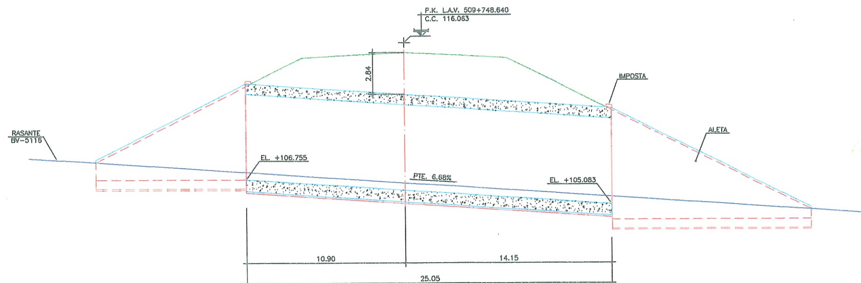
SECCIÓN A-A ESCALA 1/250
