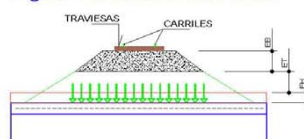
Figura 1-c: Sección transversal
