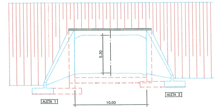
VISTA POR -B- ESCALA 1/250
