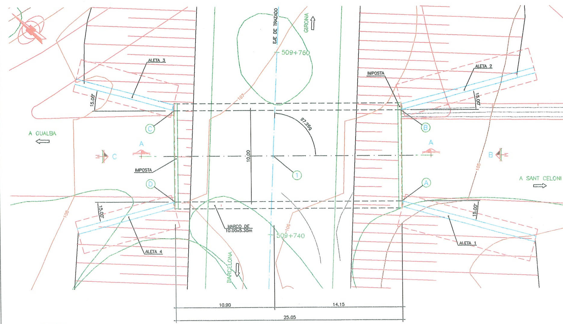
PLANTA ESCALA 1/250
