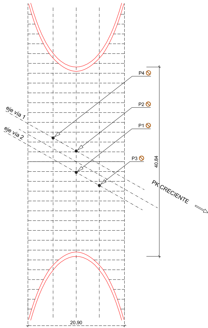
PLANTA
