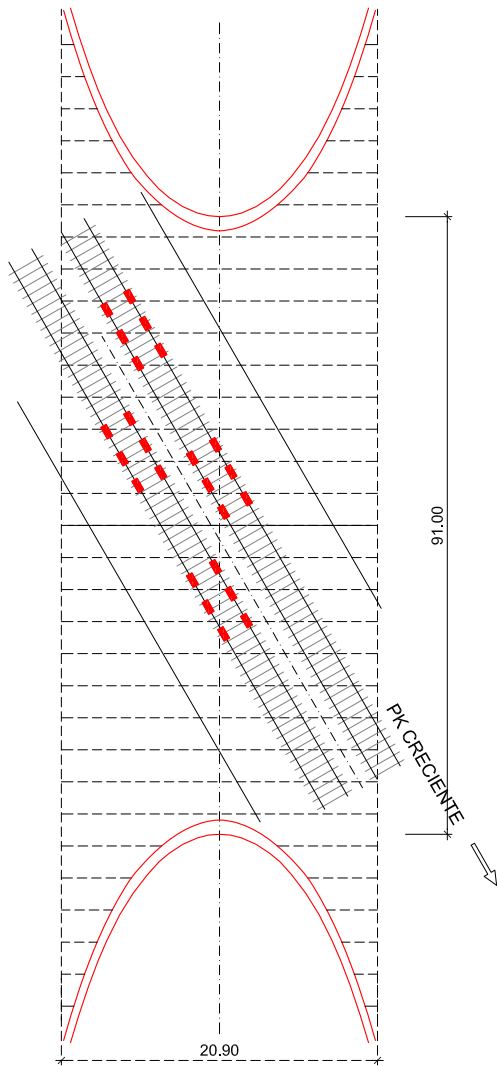
PLANTA
