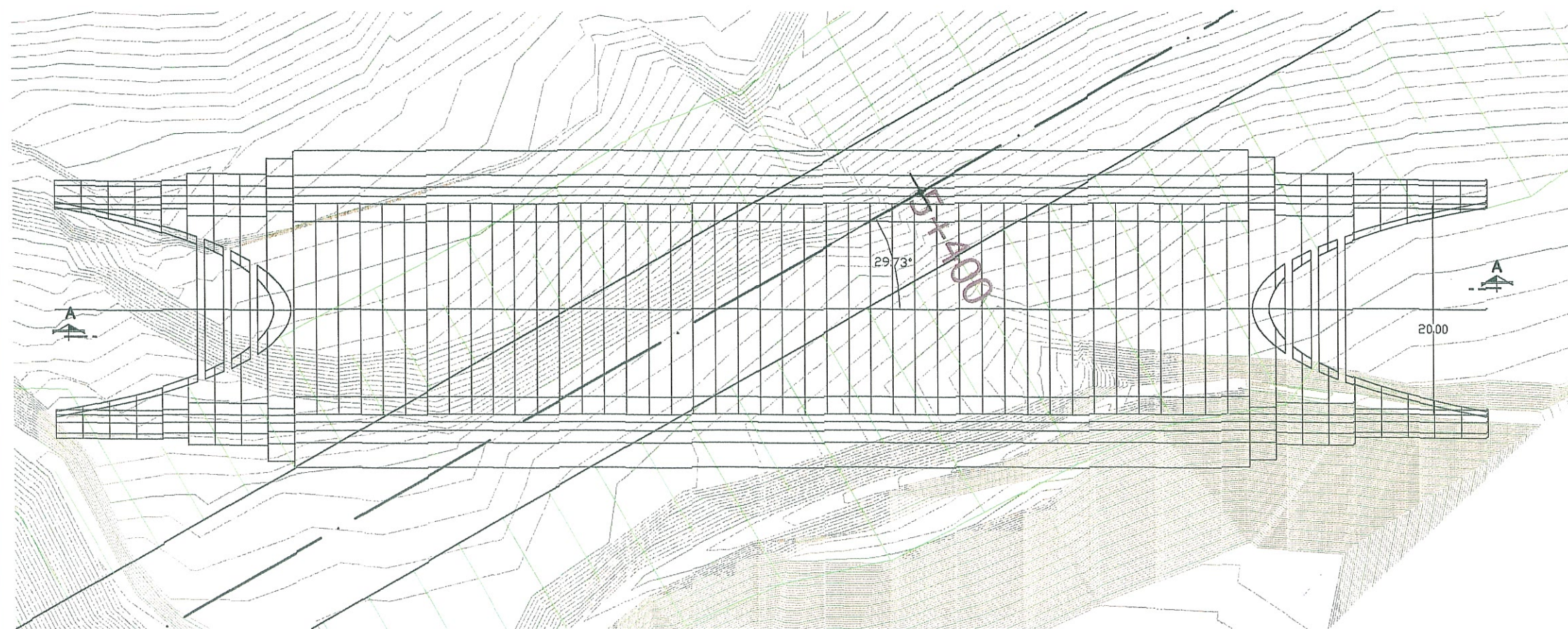
PLANTA ESCALA 1/500
