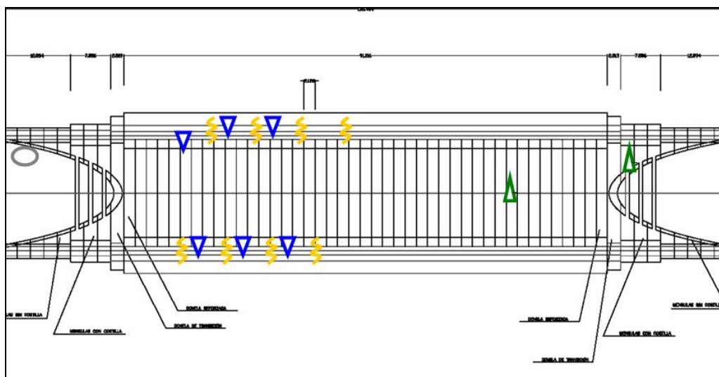
Planta.
