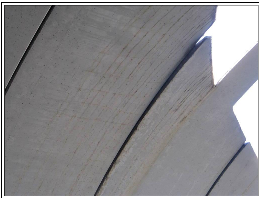
Desplazamiento de dovela con costilla.
