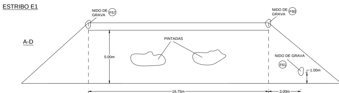
Croquis nº 1. Estribo de entrada
