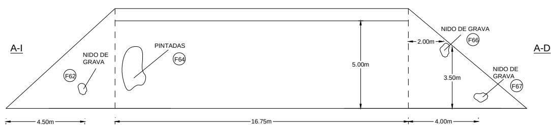
Croquis nº 2. Estribo de salida
