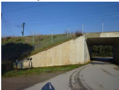
Fotografía nº 5. Estribo de entrada
