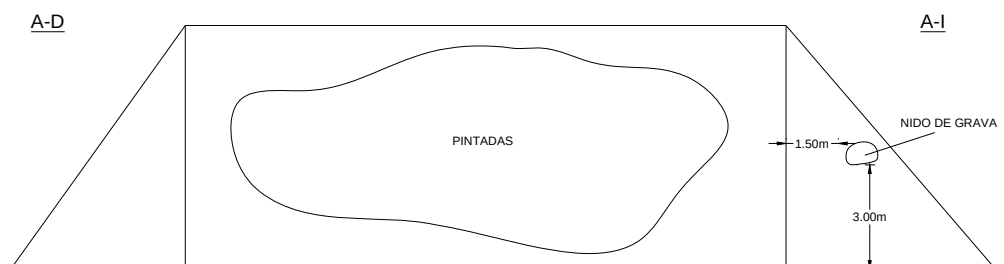
Croquis nº 1. Estribo de entrada de la obra de drenaje
