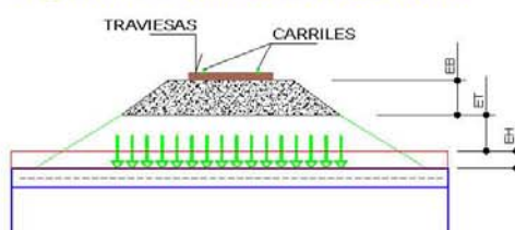
Figura 1-c: Sección transversal
