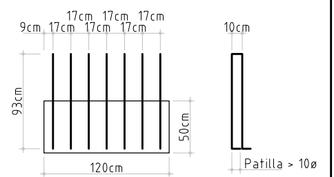
SECCIÓN A-A (DINTEL)
