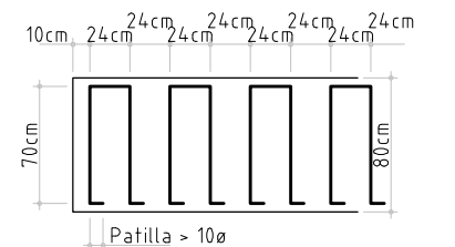
SECCIÓN D-D (CIMENTO)
