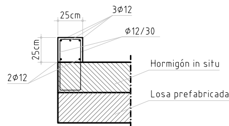
DETALLE DEL PETO
