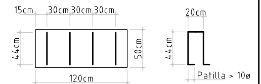
SECCIÓN B-B (HASTIAL)
