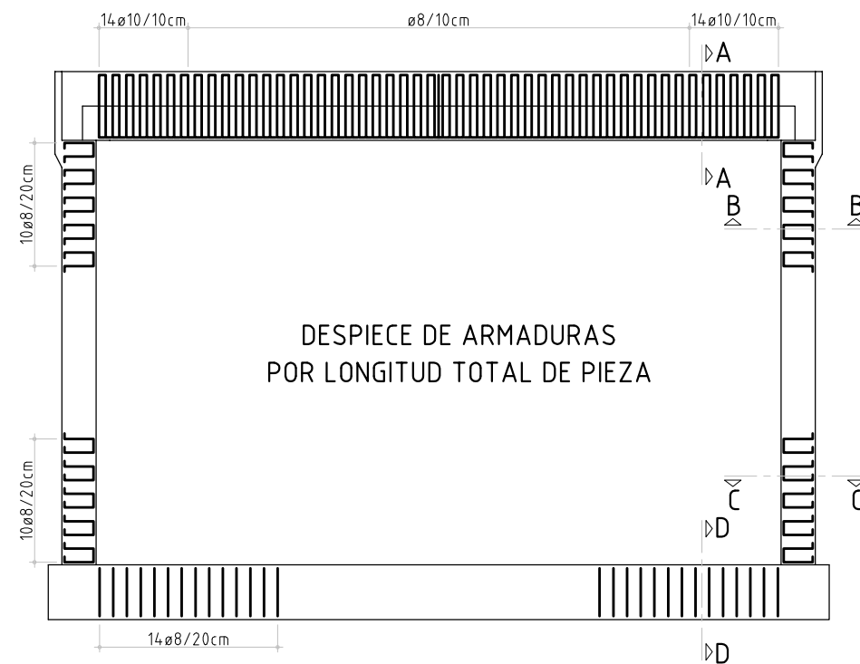
DISPOSICIÓN DE LA ARMADURA DE CORTANTE EN LOSA PREFABRICADA PASO 10X6 FA6.65 2.50x2.50 FA9.10
