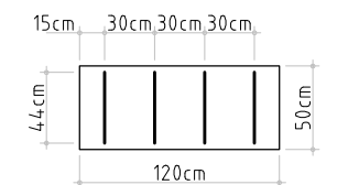
SECCIÓN C-C (HASTIAL)
