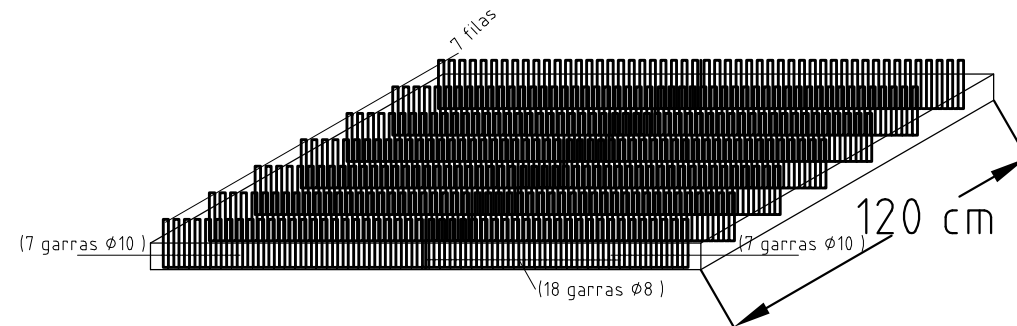
DISPOSICIÓN DE LA ARMADURA DE CORTANTE EN LOSA PREFABRICADA PASO 10X6 FA6.65 2.50x2.50 FA9.10
