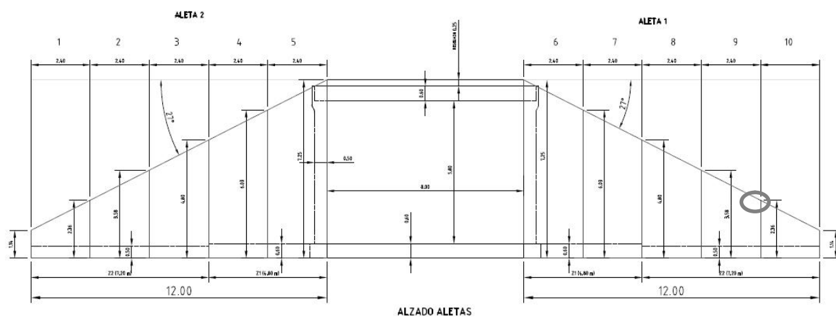
Alzado izquierdo
