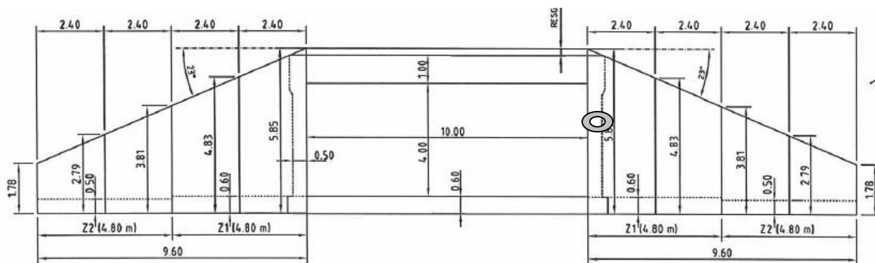
Alzado derecho
