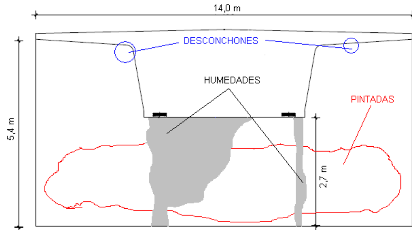
Croquis nº 5: Muro de frente del estribo de salida
