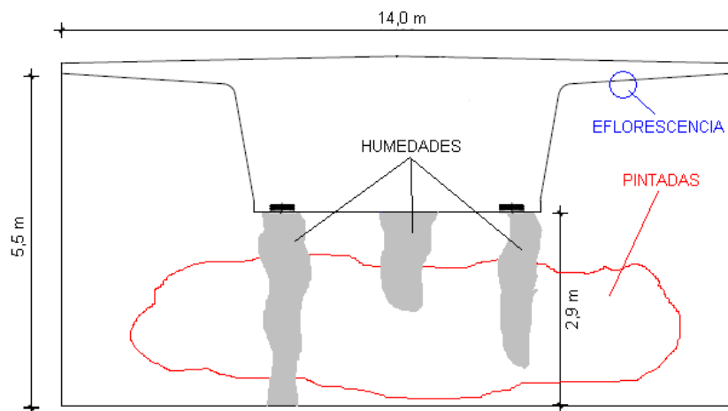
Croquis nº 4: Muro de frente del estribo de entrada
