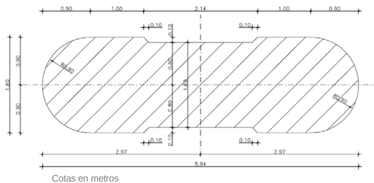
Croquis nº 3: Sección de la pila
