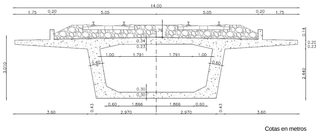
Croquis nº 2: Sección transversal del tablero
